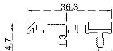
برواز الرقم التسلسلي للصنف: BLT3770 الوزن 0.224:(Kg/m)
