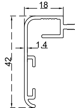
برواز سموي الرقم التسلسلي للصنف: BLT399 الوزن 0.259:(Kg/m)
