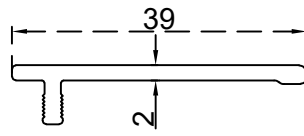
برواز مستقيم كبس 39 ملم الرقم التسلسلي للصنف: BLT868 الوزن 0.254:(Kg/m)
