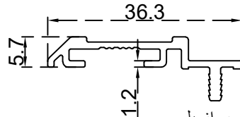
برواز بلجي الرقم التسلسلي للصنف: BLT760 الوزن 0.235:(Kg/m)
