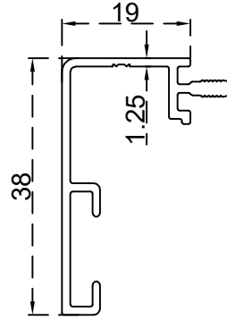
برواز عجول كبس (19*38) ملم الرقم التسلسلي للصنف: BLT3308 الوزن 0.314:(Kg/m)
