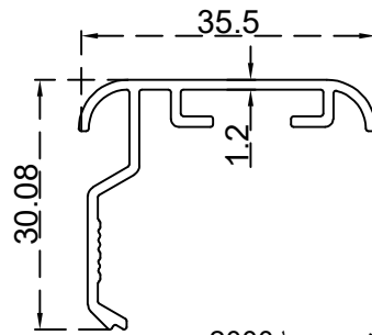
برواز سموي 2000 الرقم التسلسلي للصنف: BLT1649 الوزن 0.309:(Kg/m)
