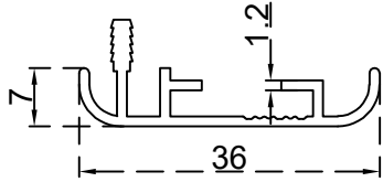
برواز كبس 36 ملم الرقم التسلسلي للصنف: BLT040 الوزن 0.251:(Kg/m)
