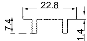
تي دبل الرقم التسلسلي للصنف: BLT031 الوزن 0.158:(Kg/m)
