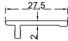
برواز مستقيم كبس 27.5 ملم الرقم التسلسلي للصنف: BLT869 الوزن 0.190:(Kg/m)
