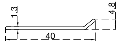
اف ماييم (5*40) ملم الرقم التسلسلي للصنف: BLT4419 الوزن 0.145:(Kg/m)
