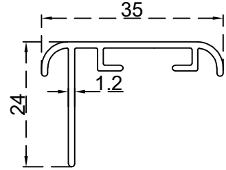
برواز سموي الرقم التسلسلي للصنف: BLT399 الوزن 0.259:(Kg/m)
