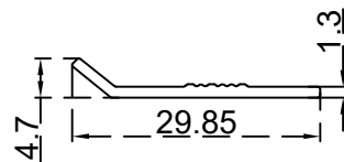
اف ماييم (5*30) ملم الرقم التسلسلي للصنف: BLT3322 الوزن 0.113:(Kg/m)
