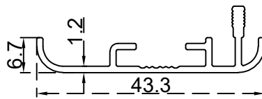
برواز كبس 43 ملم الرقم التسلسلي للصنف: BLT4782 الوزن 0.271:(Kg/m)
