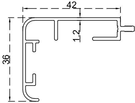
برواز عجول كبس (36*42) ملم الرقم التسلسلي للصنف: BLT3534 الوزن 0.454:(Kg/m)
