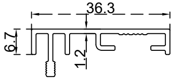
برواز مستقيم كبس 36 ملم الرقم التسلسلي للصنف: BLT4020 الوزن 0.263:(Kg/m)
